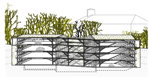
Schnitt A - A
